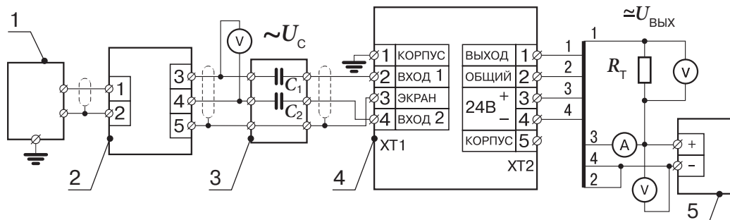
Рис. П.2. Схема соединений устройств для измерения технических характеристик УС СИЭЛ–1652–..., СИЭЛ–1654–..., СИЭЛ–1656–...
