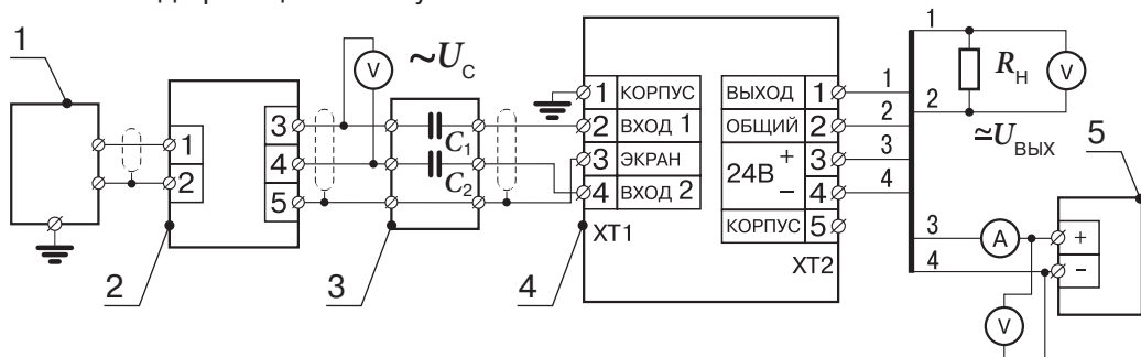
Рис. П.1. Схема соединений устройств для измерения технических характеристик УС СИЭЛ–1651–..., СИЭЛ–1653–..., СИЭЛ–1655–...
