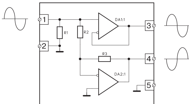
Рис. П.4. Рекомендуемая схема формирователя парафазного напряжения.
